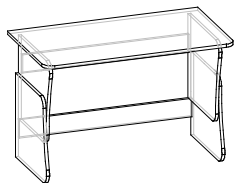
Стол 100,4 × 55,2 × 65,6* см Ширина × Глубина × Высота
