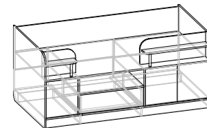
Кровать 183,2 × 95,7 × 81,2 см Ширина × Глубина × Высота Под матрас 1800x800 мм
